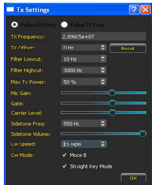
Bild 3. Tx-inställningar
