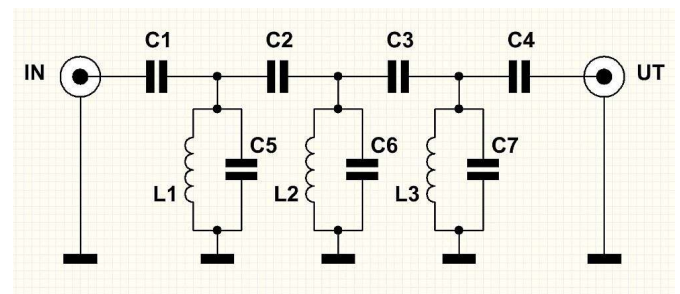
W3LPL bandpassfilter
